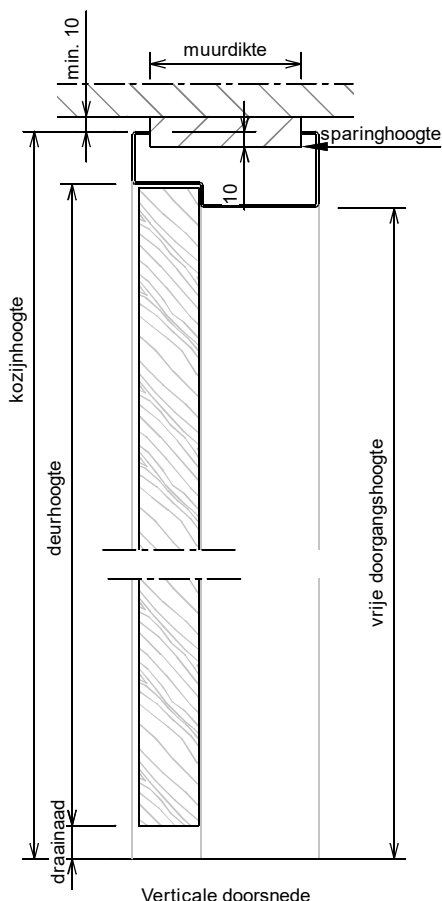
Verticale doorsnede
