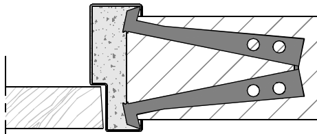
Aansluiting inmetselekozijn (+ inleganker) Optioneel: vellingblokkers
