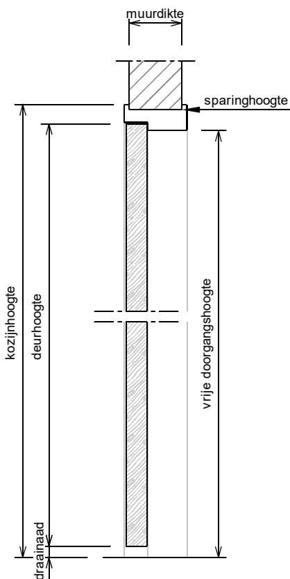
Verticale doorsnede
