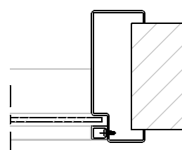
Zijlicht: Uitvoering met aluminium glaslijst 13 x 15 mm. Bij brandwerende versie stalen glaslijst (15 x 25)
