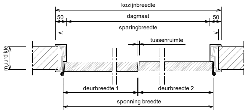
Horizontale doorsnede (uitvoering met aanslaglat of tongnaald)
