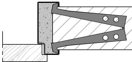
Aansluiting inmetsekozijn ( + inleganker ) Optioneel: vellingblokkers
