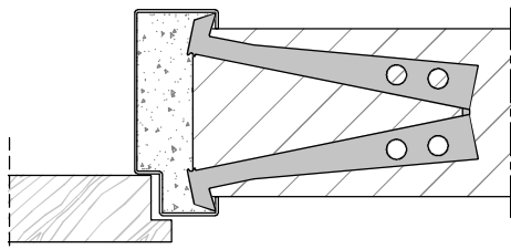
Aansluiting inmetselekozijn (+inleganker) Optioneel: Vellingblokkers
