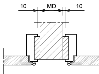
Aansluiting 2 kozijnen (losse afdeekplaat optioneel leverbaar)
