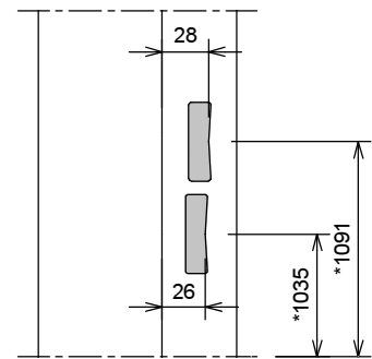
Slotgat Nef 1200-1300-1400 (optioneel)
