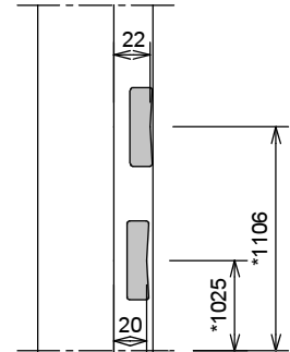
Slotgat Nemeff 600 (utiliteitsbouw)
