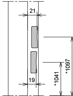
Slotgat Nemeff 1200-1300-1400 (woningbouw)
