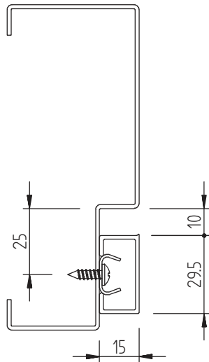
aluminium 30x15
