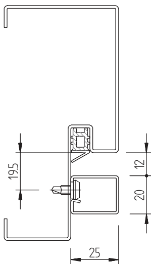
staal 20x25
