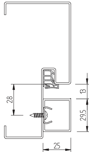
aluminium 30x25
