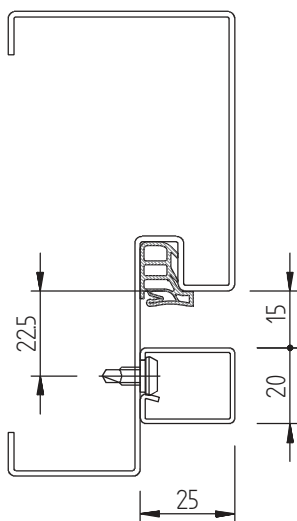
staal 20x25
