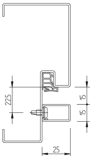
staal 15x25
