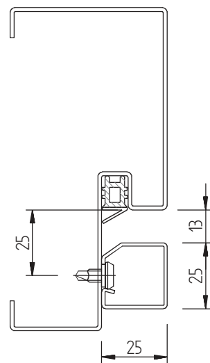
staal 25x25
