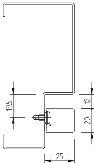
staal 20x25
