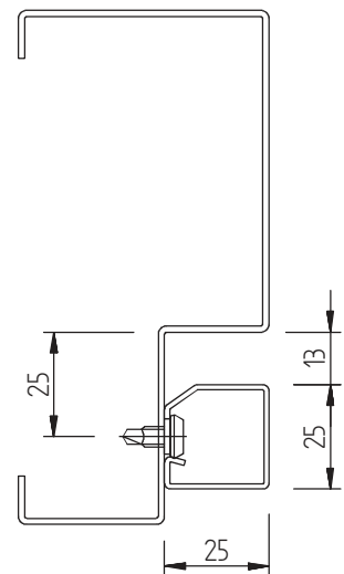
staal 25x25
