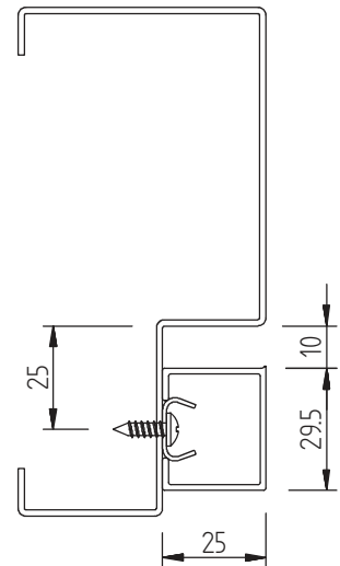
aluminium 30x25
