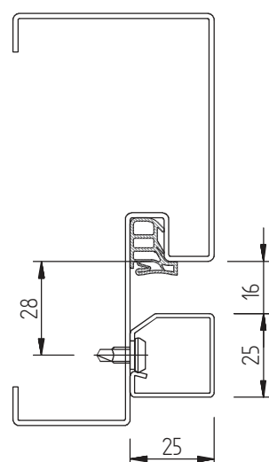
staal 25x25
