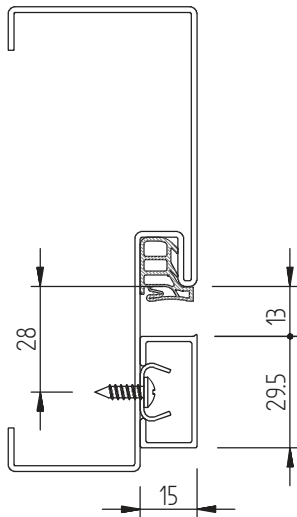
aluminium 30x15
