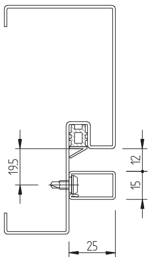
staal 15x25
