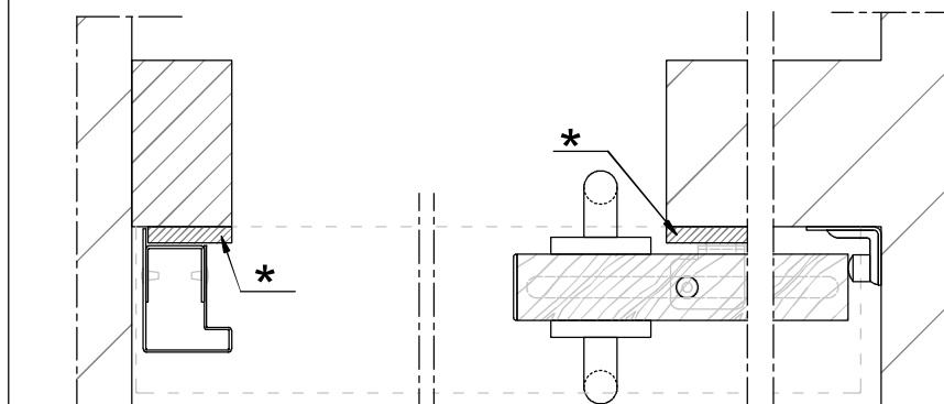
Horizontale doorsnede GV=90
