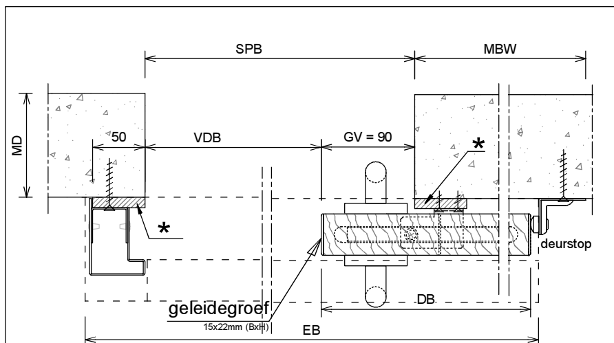
Horizontale doorsnede GV=90
