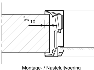
Montage- / Nasteluitvoering
