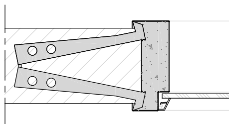
Inmetseluitvoering
