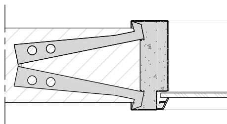
Inmetseluitvoering
