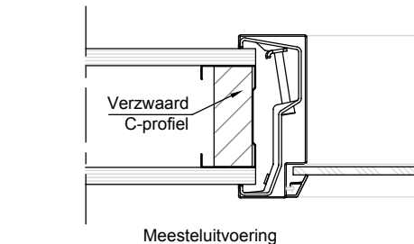
Meesteluitvoering
