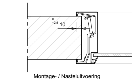
Montage- / Nasteluitvoering
