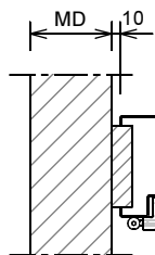
Aansluiting haakse wand
