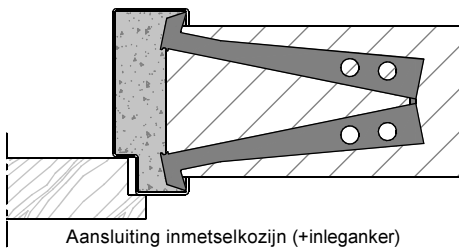
Aansluiting inmetSELkozijn (+inleganker) Optioneel: Vellingblokkankers
