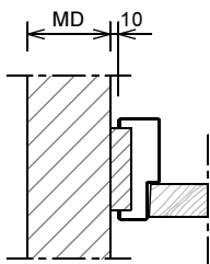
Aansluiting haakse wand
