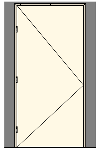
Deurdiktes 40mm en 54 mm - 3x VX7729/100 3D scharnieren
