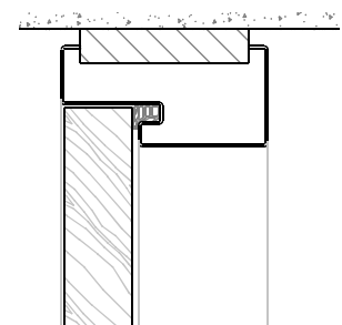
Optie: aanslagband 25 mm aanslagspinning
