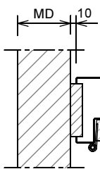
Aansluiting haakse wand
