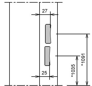
Slotgat Nemeff 1200-1300-1400 ( optioneel )
