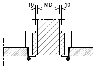
Aansluiting 2 kozijnen (losse afdeklpaat optioneel leverbaar)
