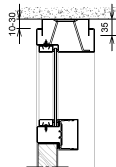
Optioneel: verende plafondregel
