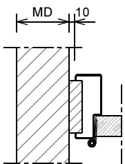
Aansluiting haakse wand
