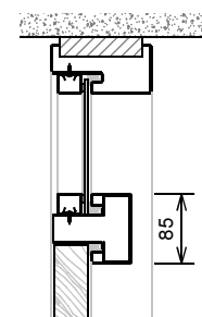
Optie: aanslagband 25 mm aanslagspanning
