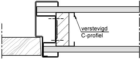
Aansluiting metalstudwand verstevigd C-profiel
