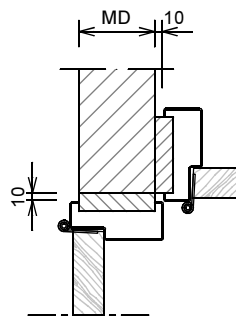
Hoekaansluiting 2 kozijnen
