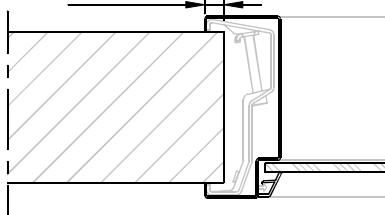
Aansluiting montagekozijn
