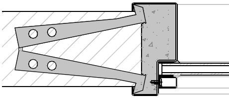
Aansluiting inmetSELuitvoering (+ inleganker) optie: veilingblokkankers
