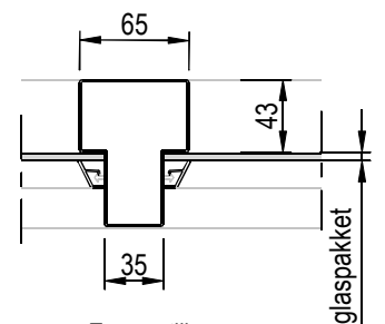
Tussenstijl
