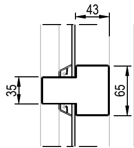
Borstwering
