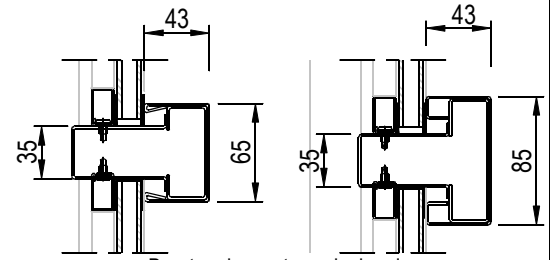
Borstwering met aanslagband sponning 15 mm sponning 25 mm
