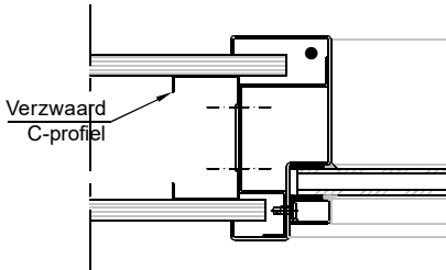
Aansluiting metalstudwand
