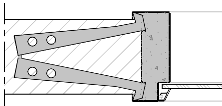
Aansluiting inmetSELuitvoering (+ inleganker) optie: veilingblokanckers
