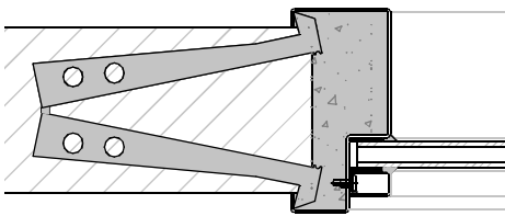
Aansluiting inmetSELuitvoering (+ inleganker) optie: veilingblokanckers
