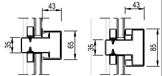
Borstwering met aanslagband spooning 15 mm spooning 25 mm
