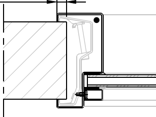
Aansluiting montagekozijn
