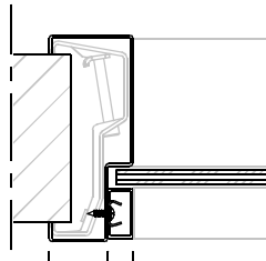
15 mm aanslagspooning aluminium glaslijst
