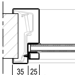
Optie: 25 mm aanslagspooning stalenglaslijst
