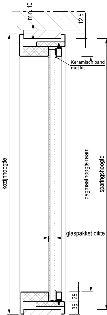
Verticale doorsnede
