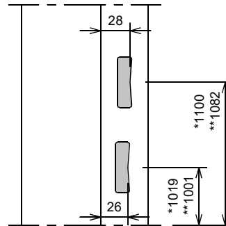
Slotgat Nemef 600
