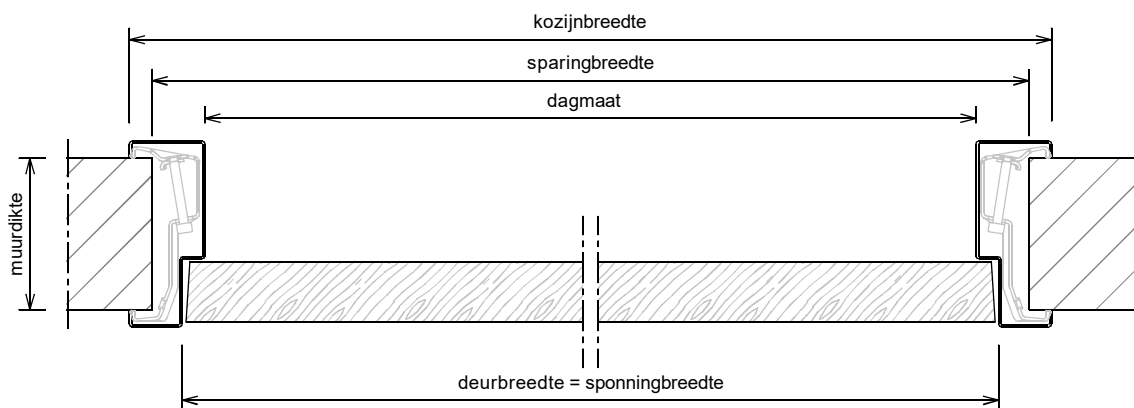
Horizontale doorsnede
