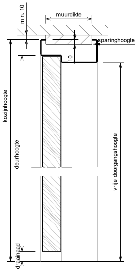
Verticale doorsnede
