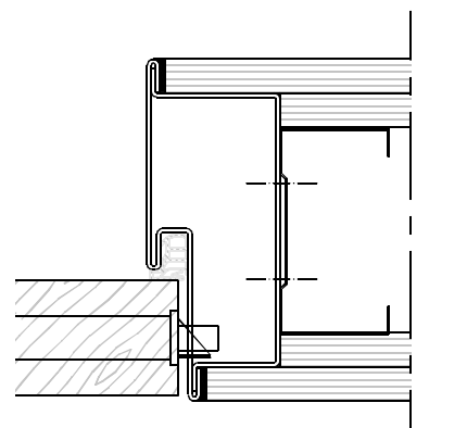
Aanslagspinning 15 mm Dubbel gips
