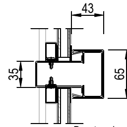
Borstwering met aanslagband sponning 15 mm
