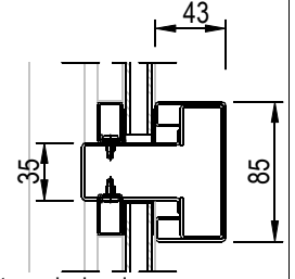
Borstwering met aanslagband sponning 15 mm
