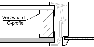
Aansluiting metalstudwand
