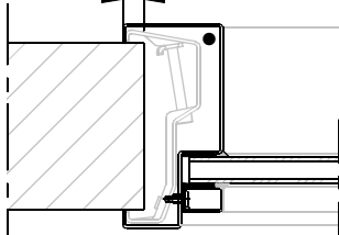
Aansluiting montagekozijn
