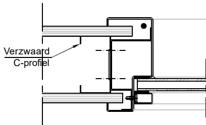
Aansluiting metalstudwand
