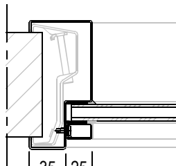
Optie: 25 mm aanslagspanning stalenglaslijst
