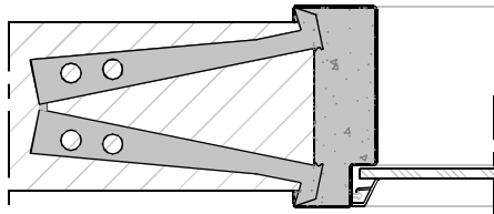
Aansluiting in metseluitvoering (+ inleganker) optie: veilingblokkankers
