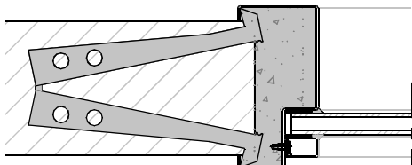
Aansluiting in metseluitvoering (+ inleganker) optie: veilingblokkankers
