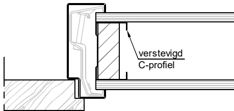
Aansluiting metalstudwand
