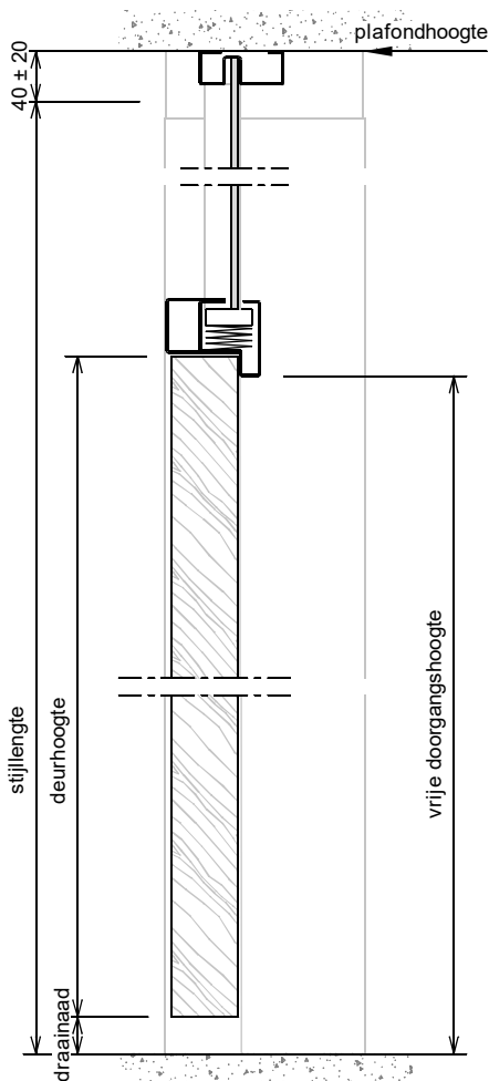
Verticale doorsnede
