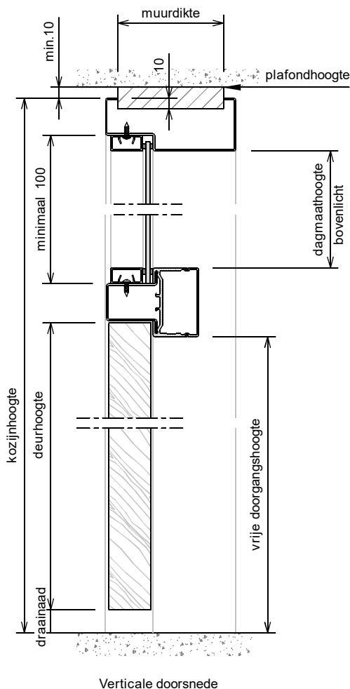
Verticale doorsnede
