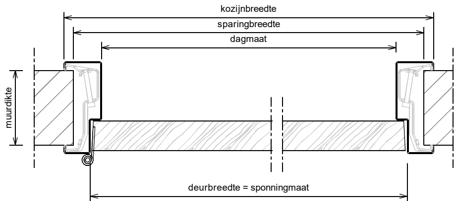
Horizontale doorsnede
