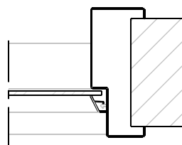
Zijlicht: Uitvoering met PVC / Kunststof glaslijst Glaspakketdikte 4 - 6 mm.
