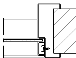
Zijlicht/ bovenlicht: Uitvoering met aluminium glaslijst 30 x 15 mm.
