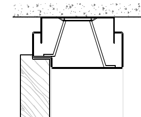
Optie: Verende plafondregel Niet bij kozijnen met zijlicht
