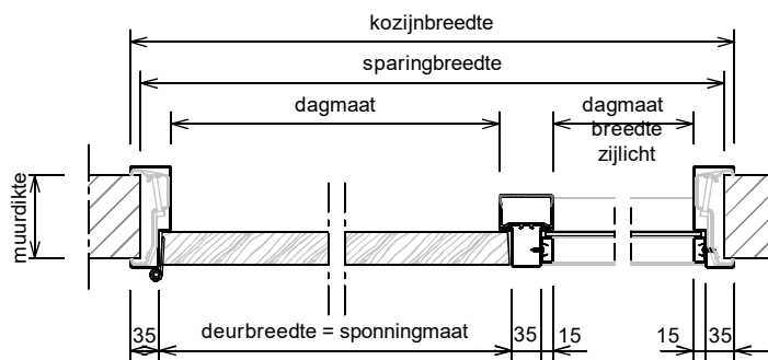
Horizontale doorsnede
