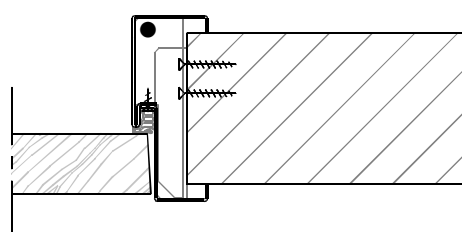
Tweeschalig kozijn (alleen aanslagband mogelijk)
