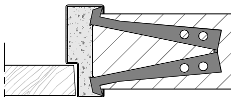
Aansluiting inmetselekozijn ( + inleganker ) Optioneel: vellingblokkankers
