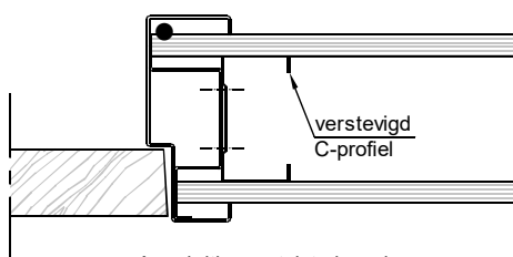
Aansluiting metalstudwand
