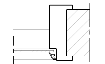
Zijlicht/ bovenlicht: Uitvoering met PVC / Kunststof glaslijst Glaspakketdikte 4 - 6 mm.
