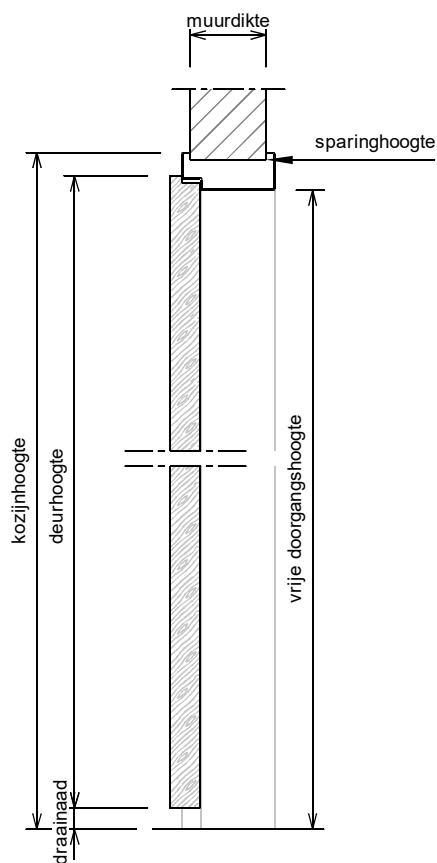
Verticale doorsnede
