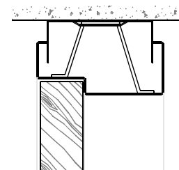
Optie: Verende plafondregel Niet bij kozijnen met zijlicht
