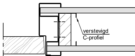
Aansluiting metalstudwand verstevigd C-profiel
