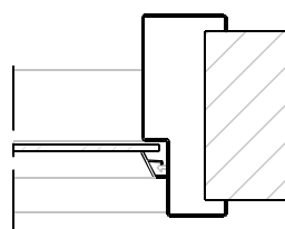
Zijlicht: Uitvoering met PVC / Kunststof glaslijst Glaspakketdikte 4 - 6 mm.
