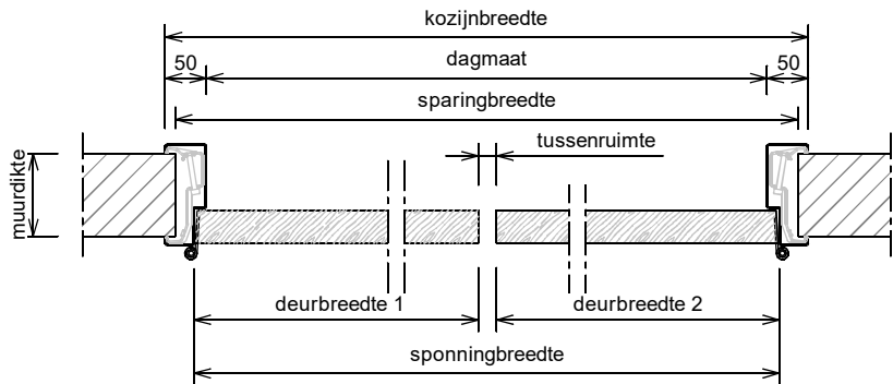
Horizontale doorsnede met tongnaald of aanslaglat
