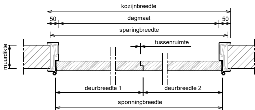
Horizontale doorsnede ( loop - stand uitvoering )
