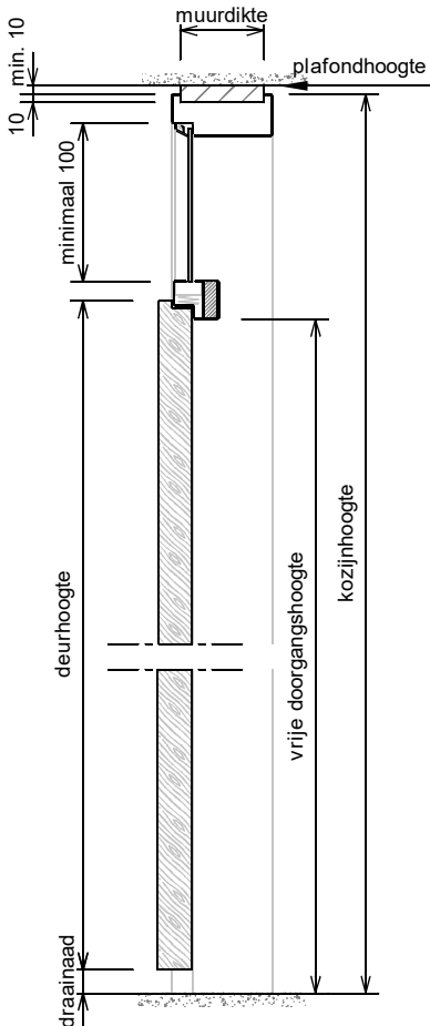
Verticale doorsnede
