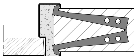
Aansluiting in metselkozijn ( + inleganker ) Optioneel: vellingblokankers
