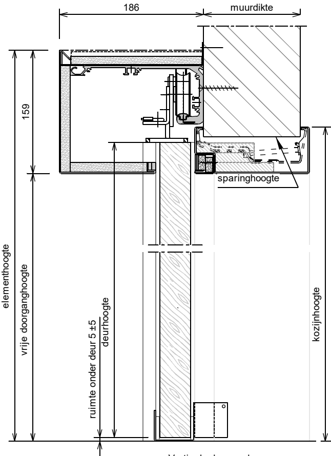
Verticale doorsnede
